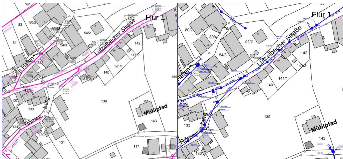
Abbildung 9: Kanalbestandsplan
